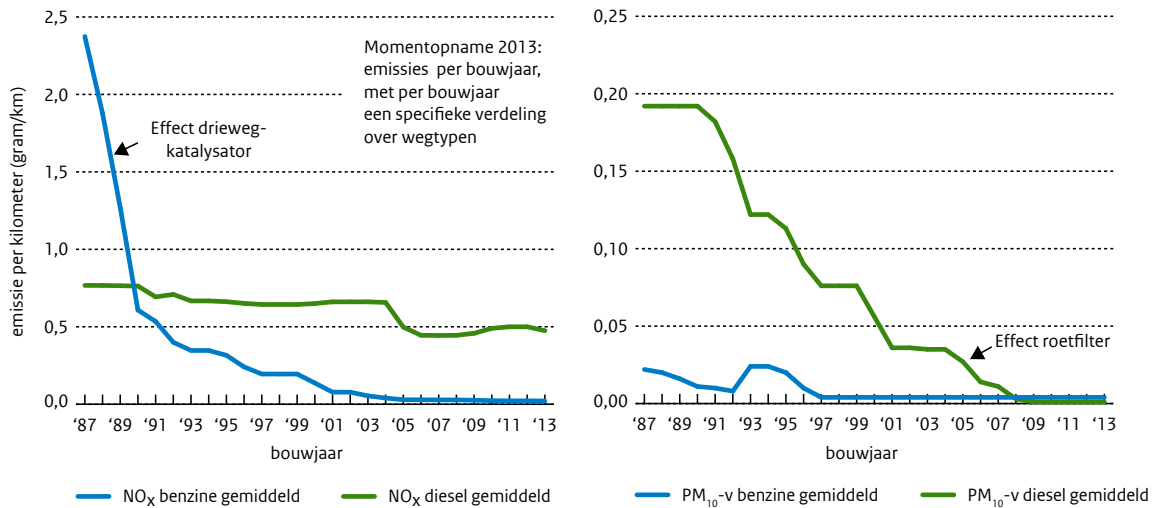
Momentopname (2013) van NO x - en PM 10 -verbrandingsemissies per kilometer van diesel- en personenauto's met de bouwjaren 1987-2013, gewogen naar het kilometrage per wegtype dat specifiek is voor elke combinatie van bouwjaar en brandstofsoort. Bron: Traa en Geilenkirchen (2013).
