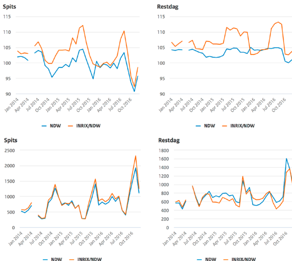
Figuur 2. Vergelijking van rijsnelheid (km/u, boven) en reistijdverlies op hoofdwegen (onder) per maand 2014-2016 tussen detectielussen (NDW) alleen en de combi van mobiele data (INRIX) en detectielussen (NDW) in de spits (7-9; 16-18 uur) en restdag. Bron: KiM.
